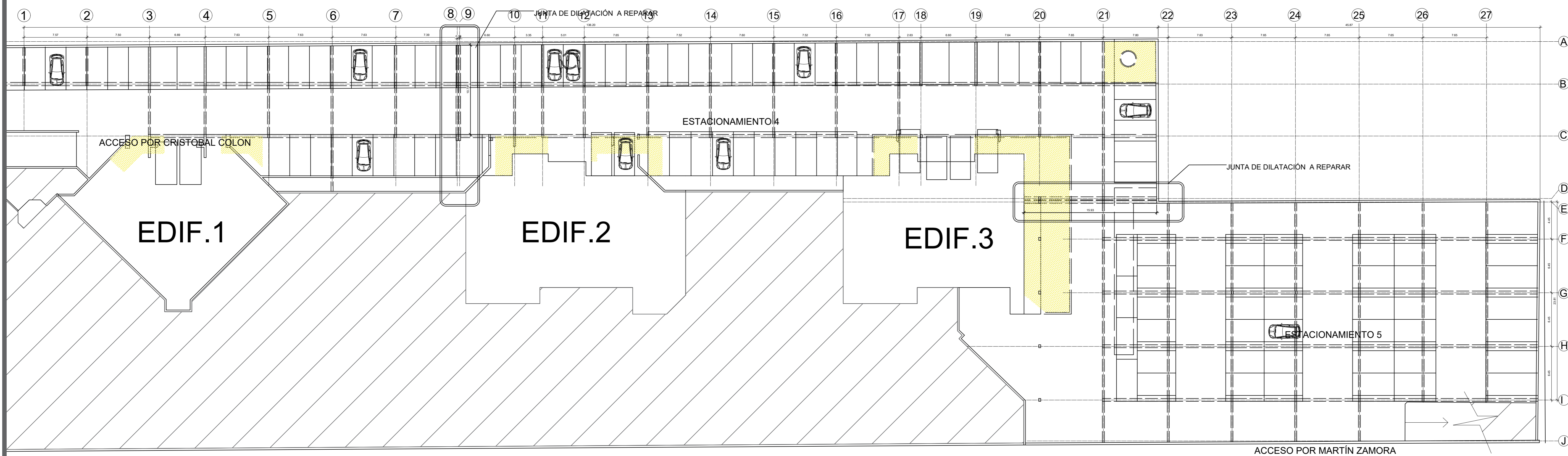
2 PLANTA CONJUNTO - NIVEL SÓTANO ESC. 1:250
